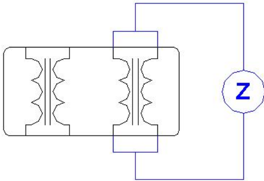
(A):Common mode
